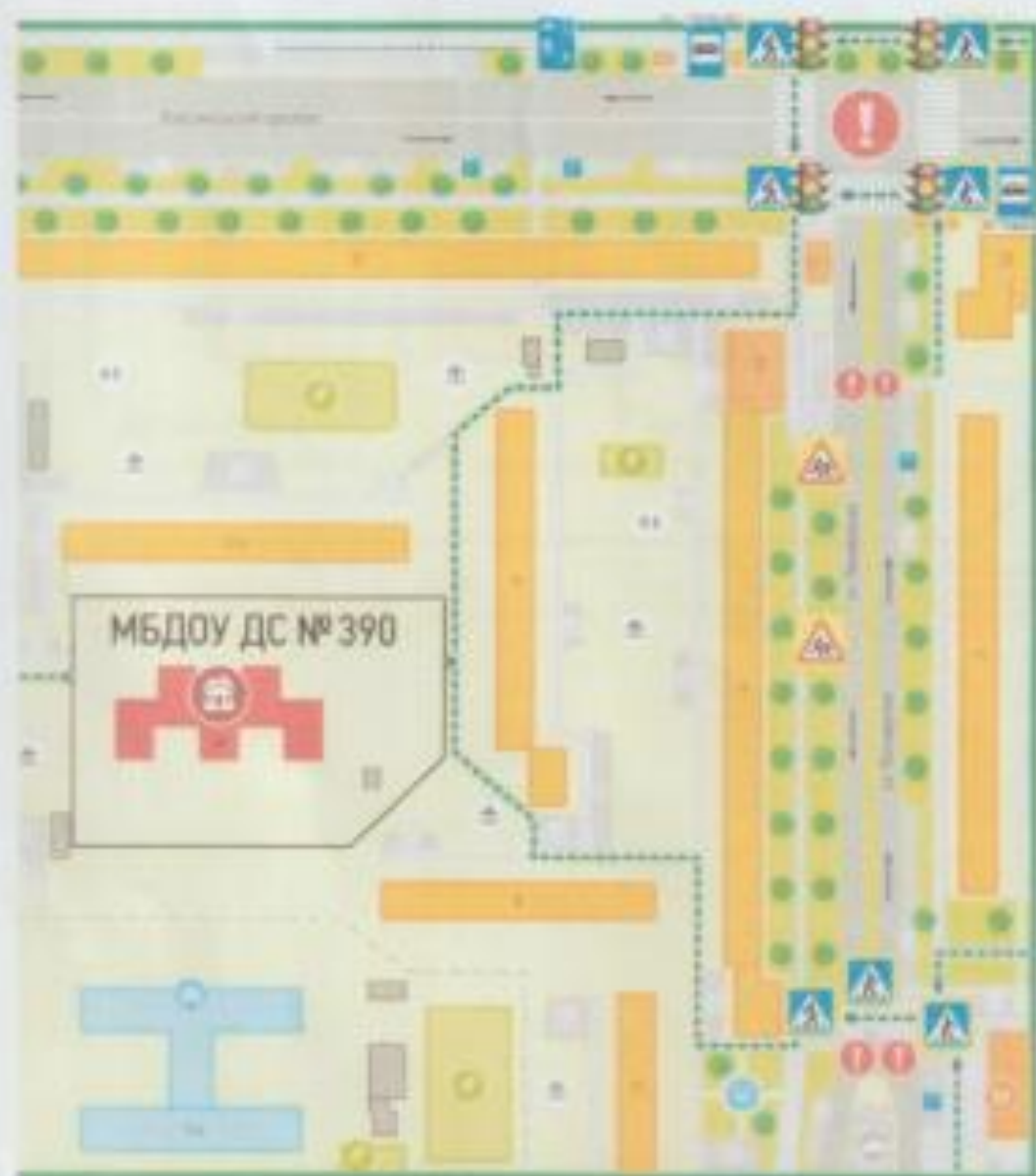
Схема 2. Организация дорожного движения в непосредственной близости от образовательного учреждения с размещением соответствующих технических средств, маршруты движения детей и расположение парковочных мест
